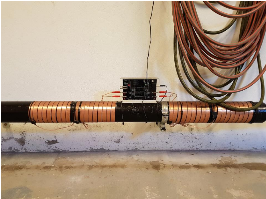
Afkalkningsanlæg
